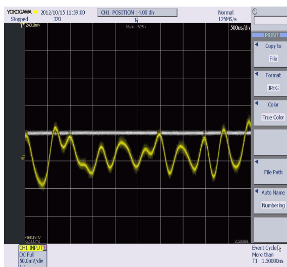
3.40 Излазни сигнал за фреквенцију 3 KHz
