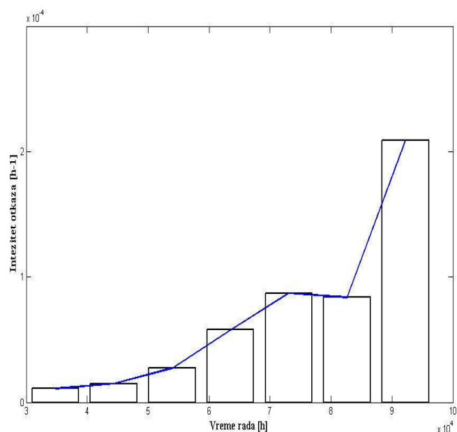
Слика 5.2 Приказ процењене функције интензитета отказа
