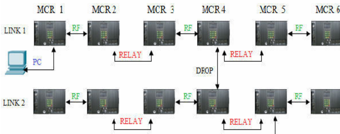
Слика 2.11 Пример мреже за надзор и управљање са PPU
