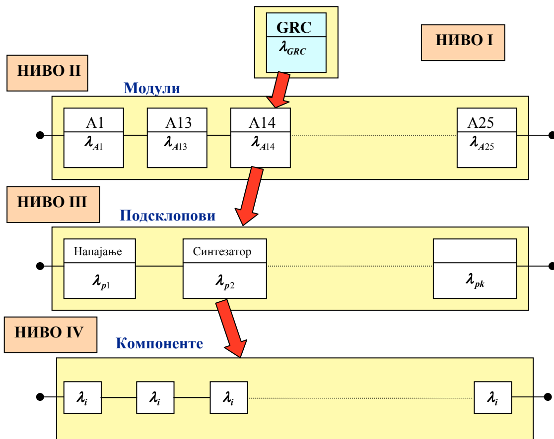
Слика 3.55 Подела RRU по функцијским и технолошким целинама
