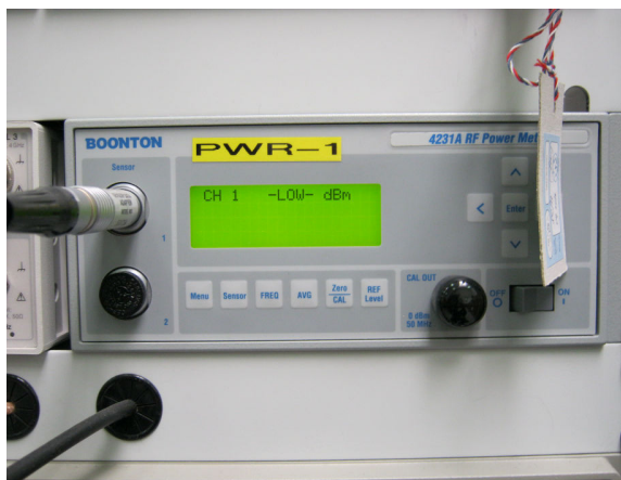
Слика 3.17 Мерач РФ снаге PWR-1 Boonton 4231A
