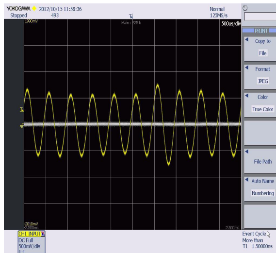
3.38 Излазни сигнал за фреквенцију 2KHz
