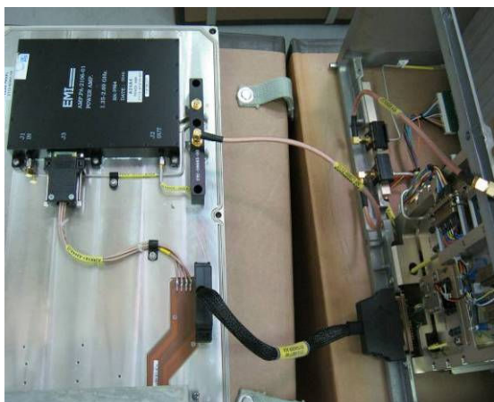
Слика 3.27 Мерење улазног сигнала у појачавач снаге
