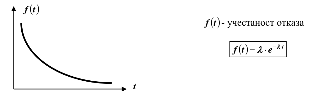
Слика 3.51 Учестаност отказа у функцији времена експоненцијалног карактера
