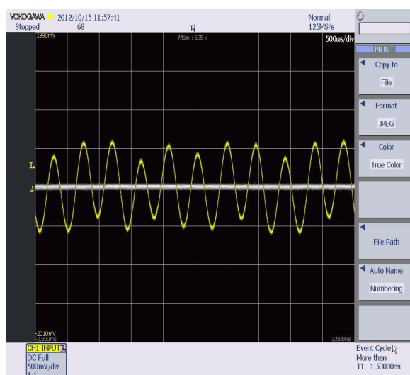
3.39 Излазни сигнал за фреквенцију 2,2 KHz
