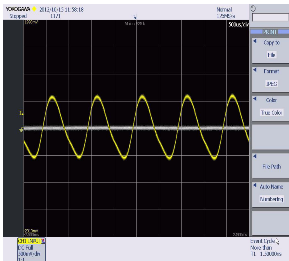
3.37 Излазни сигнал за фреквенцију 1 KHz
