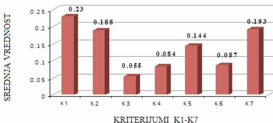
Слика 4.10 Графички приказ поретка критеријума у моделу
