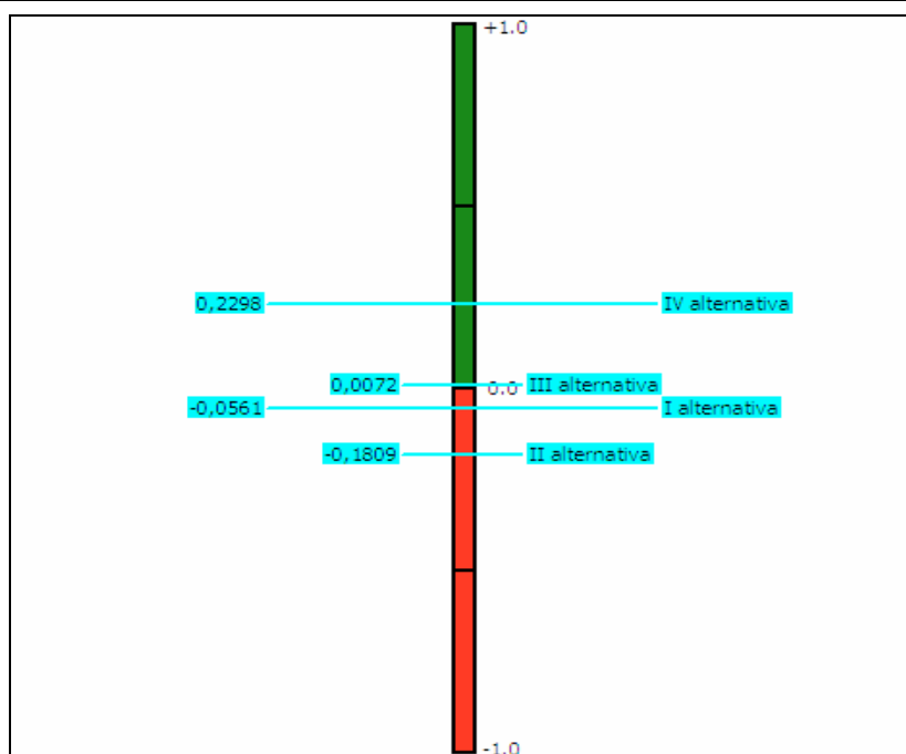
Слика 4.7 Вредност чистих токова и ранг алтернатива
