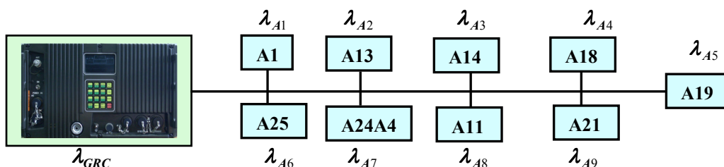
Слика 3.54 Распоред интензитета отказа по саставним модулима
