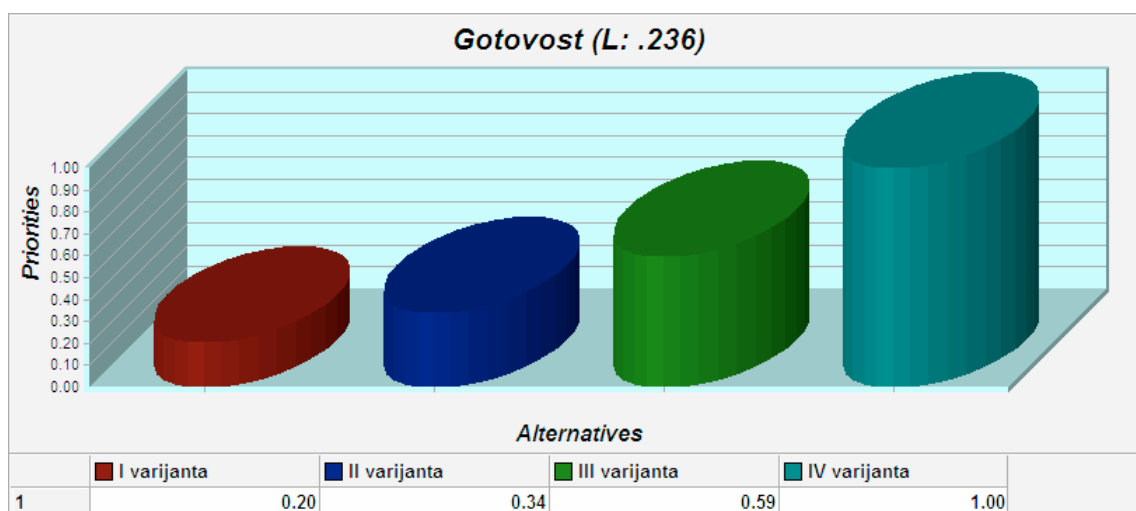
Слика 4.14 Поређење варијанти у односу на доминатан критеријум K1
