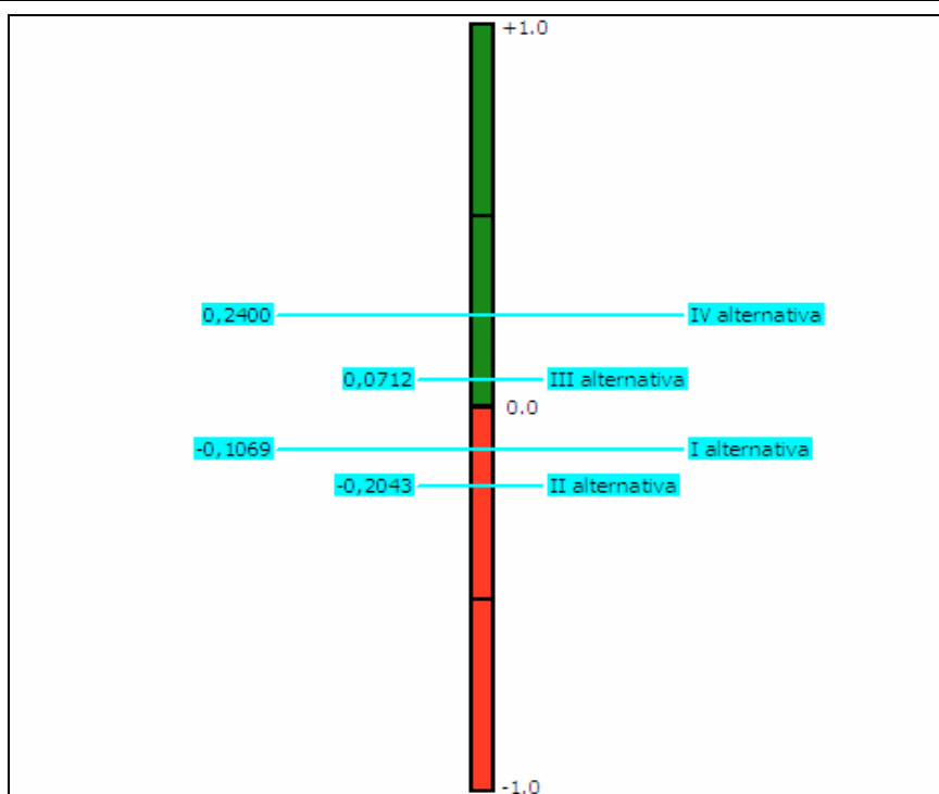
Слика 4.17 Графички приказ ранга алтернатива по методи PROMETHEE II
