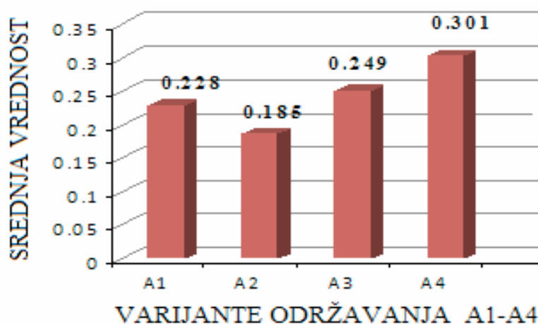
Слика 4.11 Коначни ранг варијанти организације одржавања
