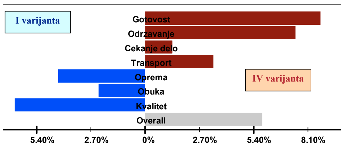
Слика 4.16 Међусобно поређење доминатних варијанти одржавања
